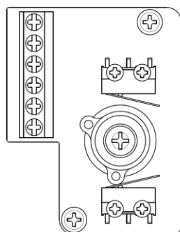
<机械式开关模块>
