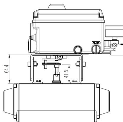
<叉型反馈杆的安装例图>
