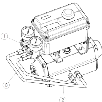
<角行程双作用>
