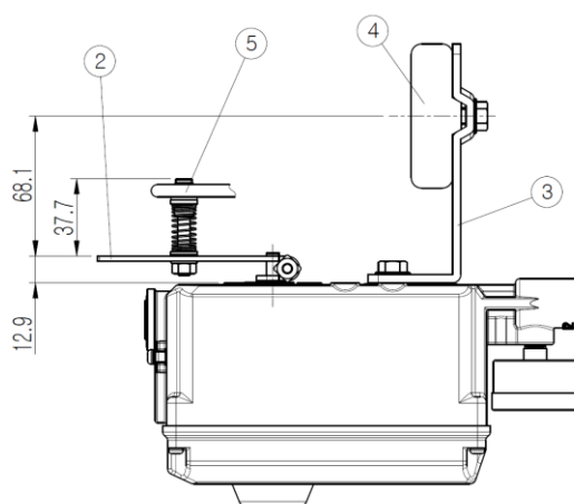
<1,2 号反馈杆>
