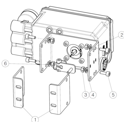
<叉型反馈杆>
