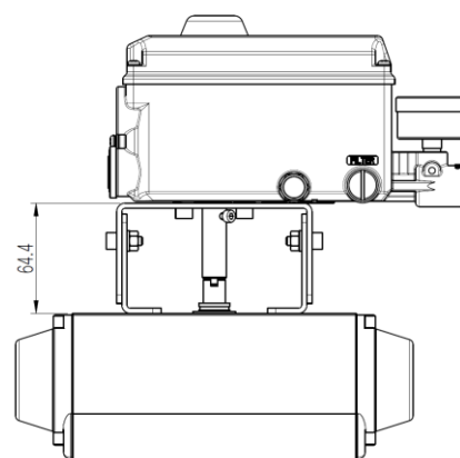
<NAMUR 型反馈杆的安装例图>
