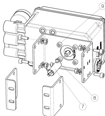
<NAMUR 型反馈杆>
