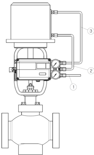
<直行程双作用型>
