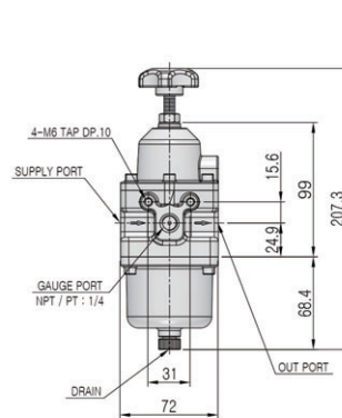
TS310/315 MANUAL DRAIN
